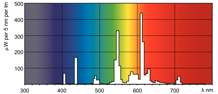
Işık rengi /827
