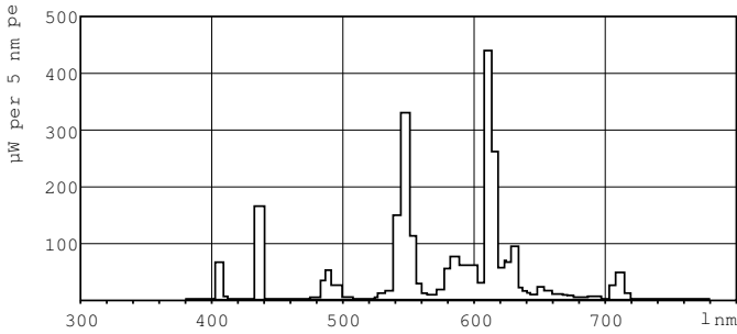
Işık rengi /827
