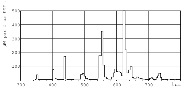
Işık rengi /827
